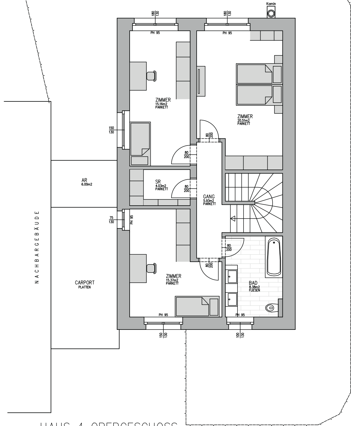
HAUS 4 OBERGESCHOSS
