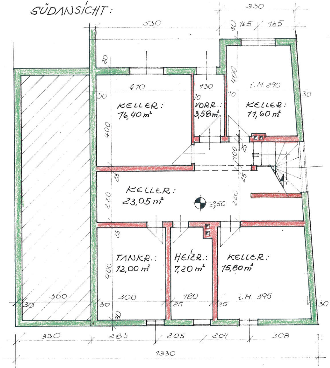
KELLERGE SCHOSS :
