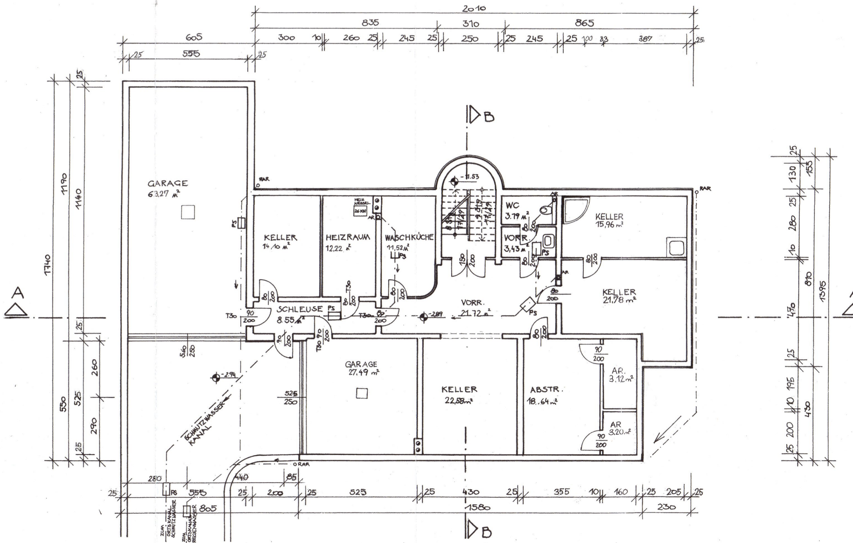
2. KELLERGESCHOSS
