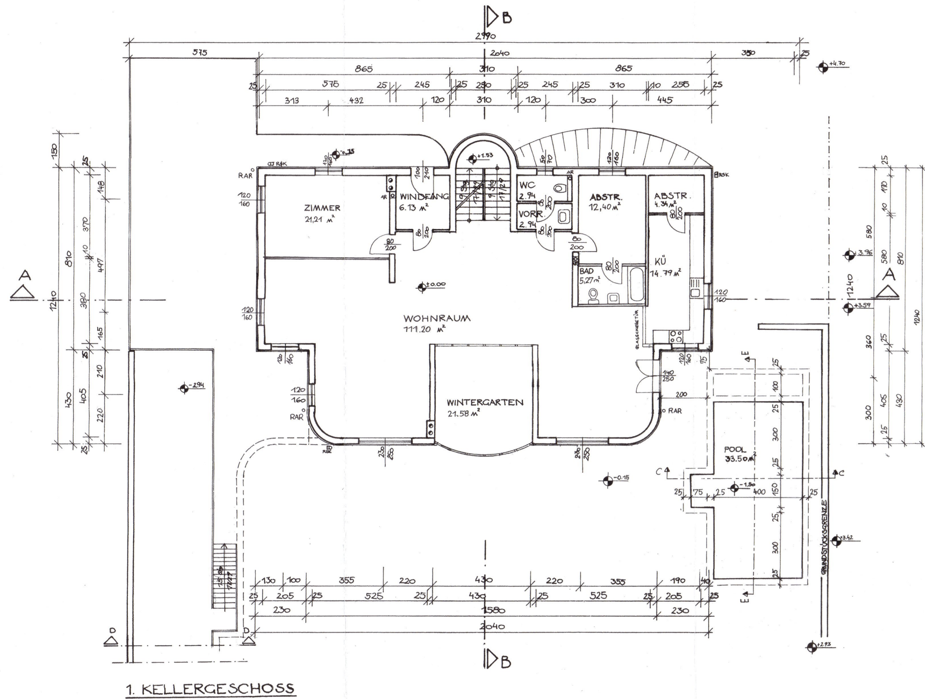
1. KELLERGESCHOSS
