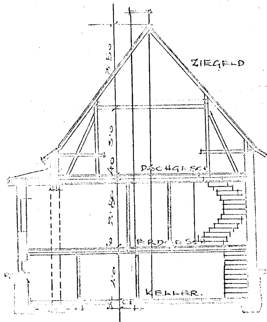
Schnitt
