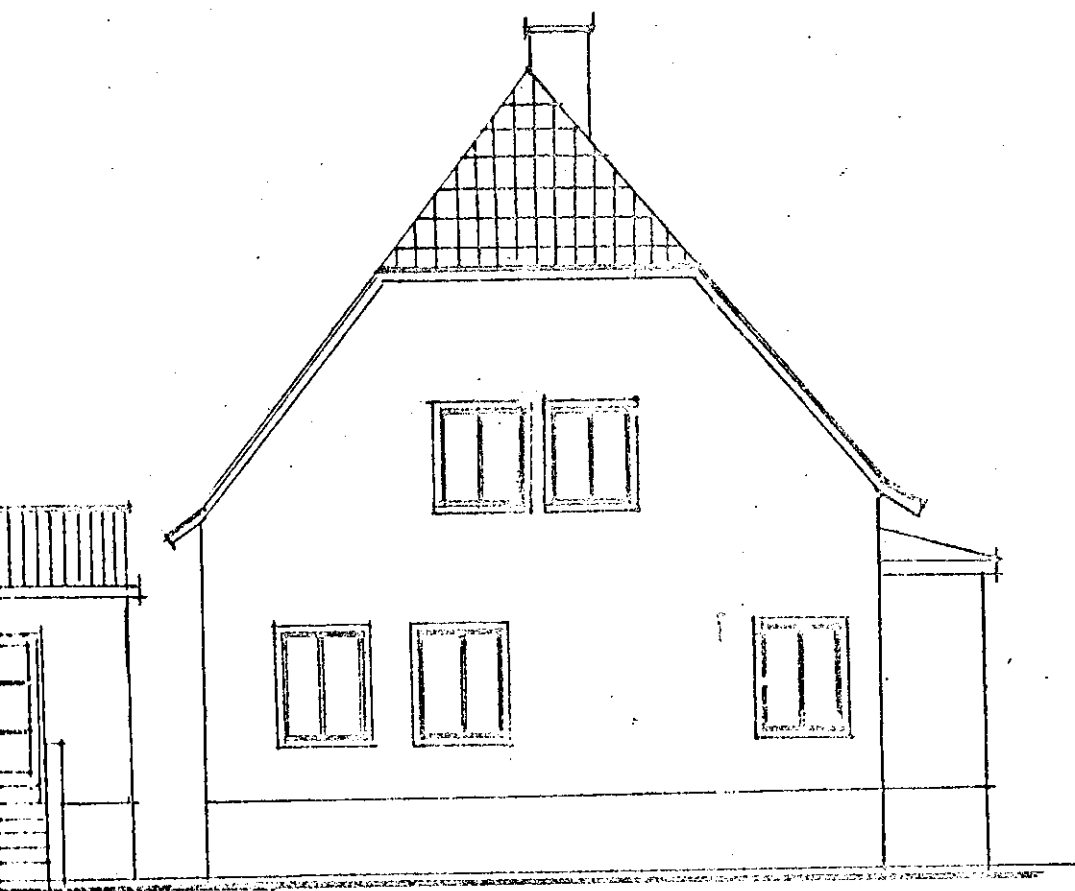
West-Ansicht
