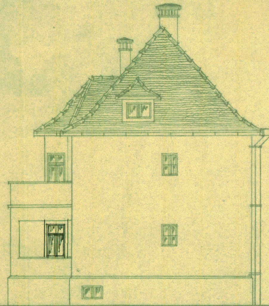
Südwest
