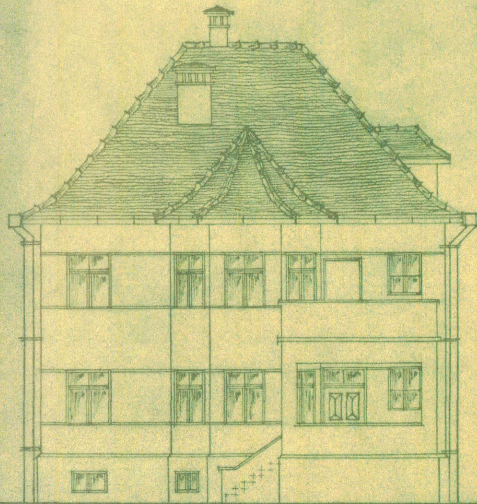
Ansicht-Nordwest
