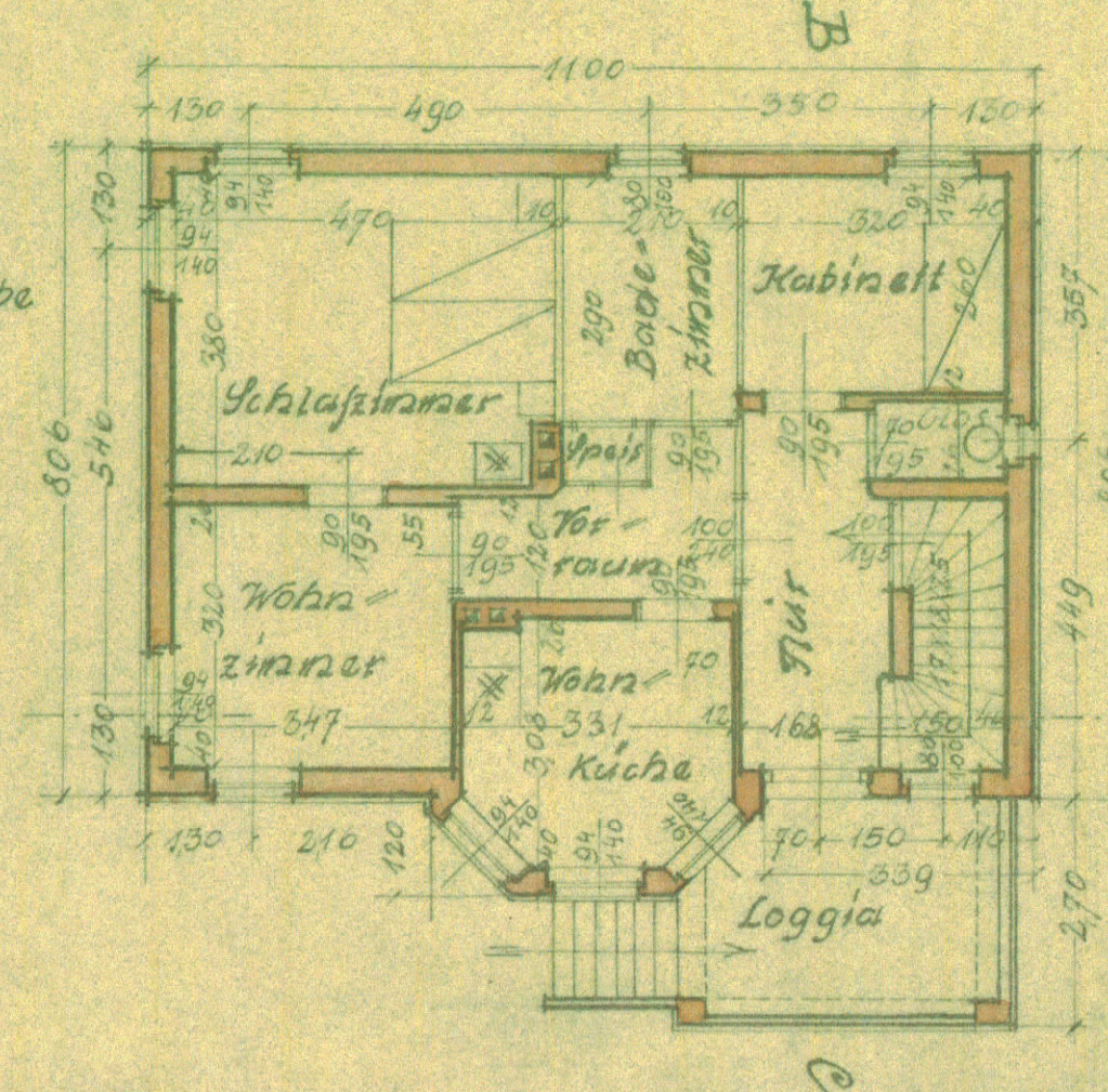
Parterregrundriss
