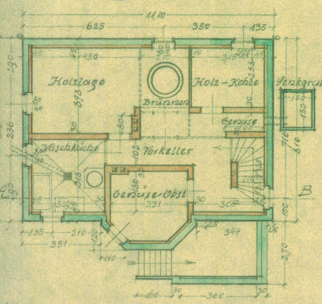
Kellergrundriss
