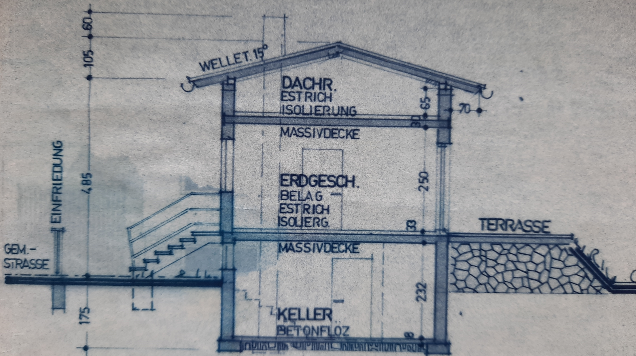
QUERSCHNITT
