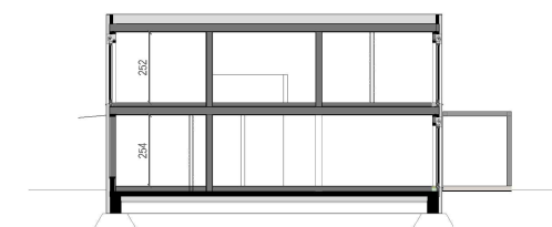
SCHEMATISCHER SCHNITT M 1:300
