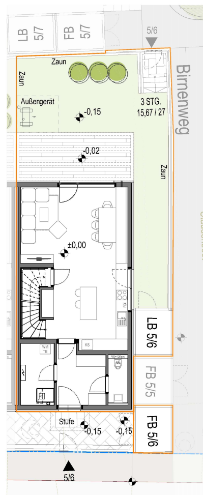
ERDGESCHOSS
