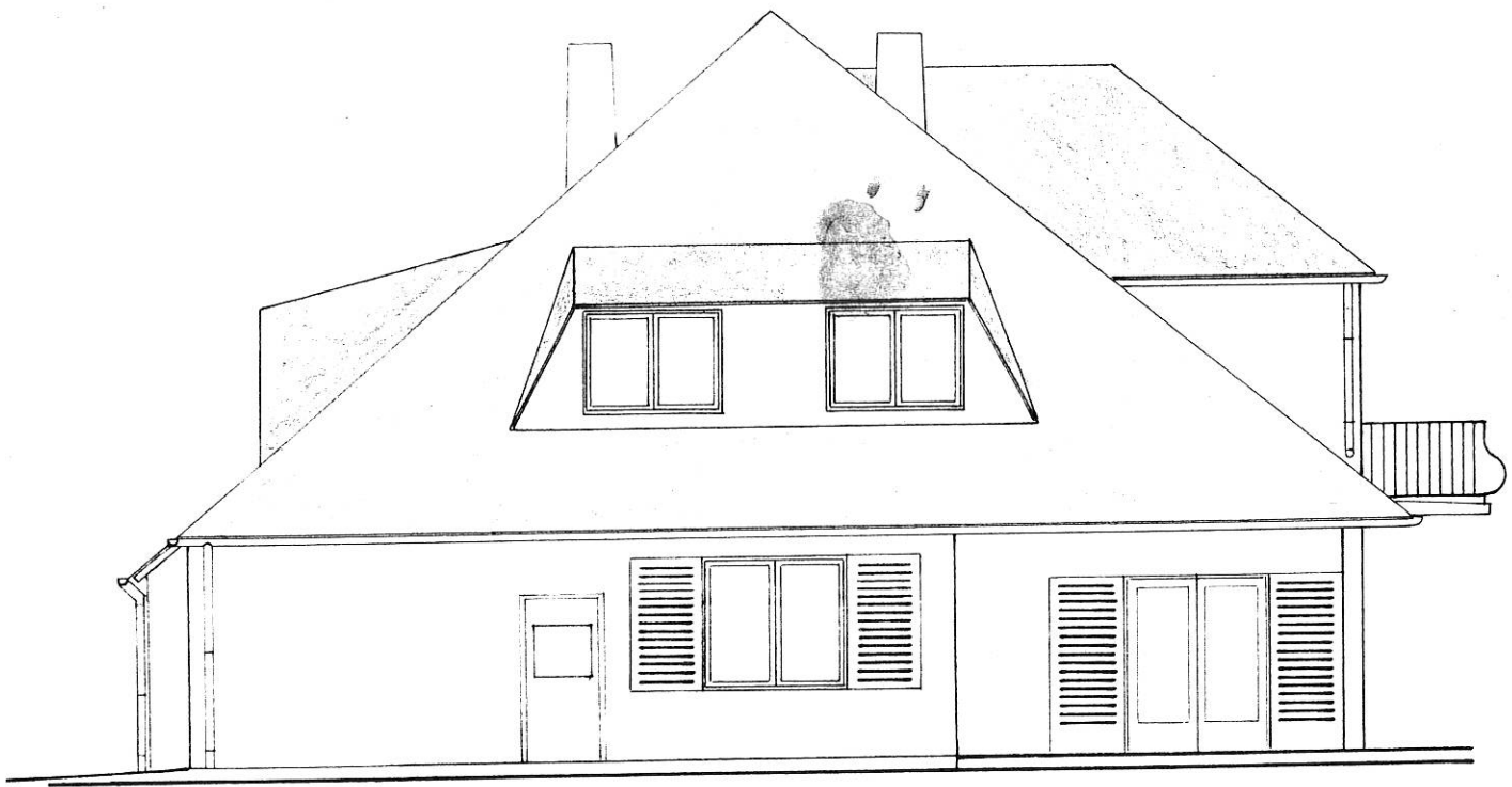
SÜDANSICHT
