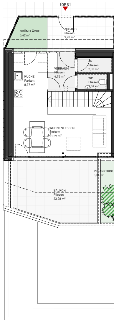
1tes OBERGESCHOSS
