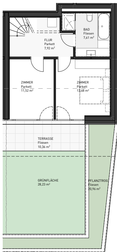
ERDGESCHOSS
