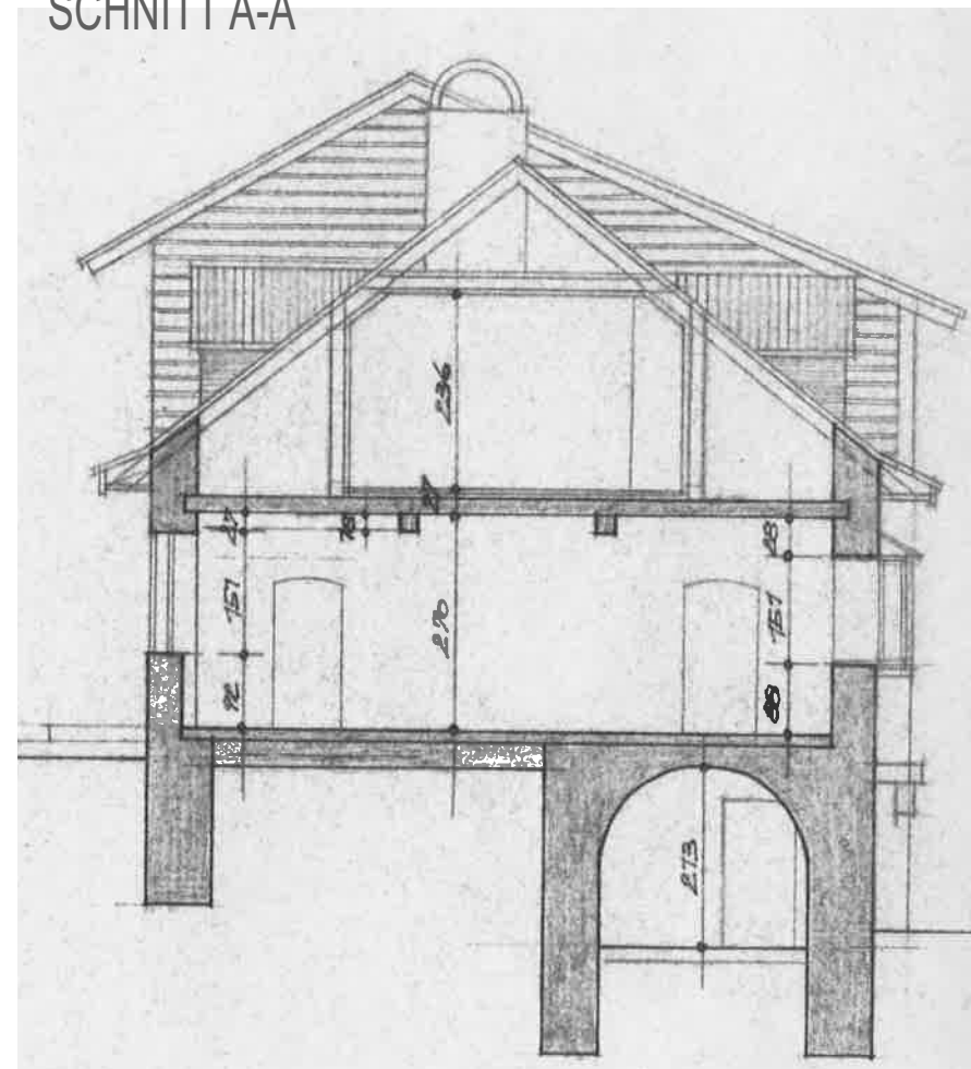
SCHNITT A-A
