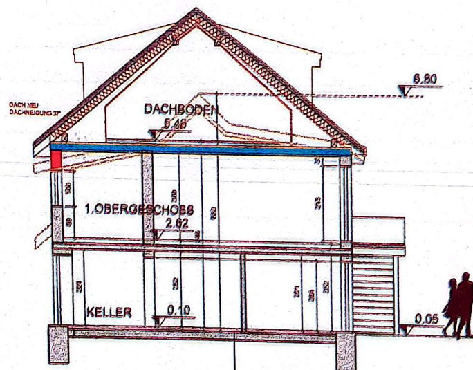
SCHNITT 3-3
