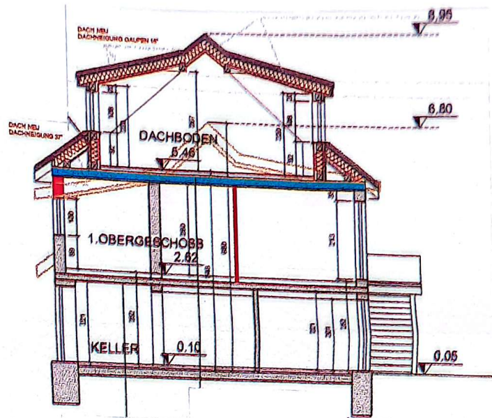
SCHNITT 2-2 GAUPEN
