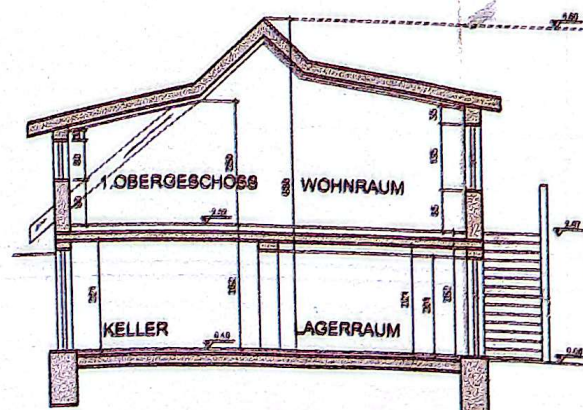
SCHNITT 1-1 BESTAND
