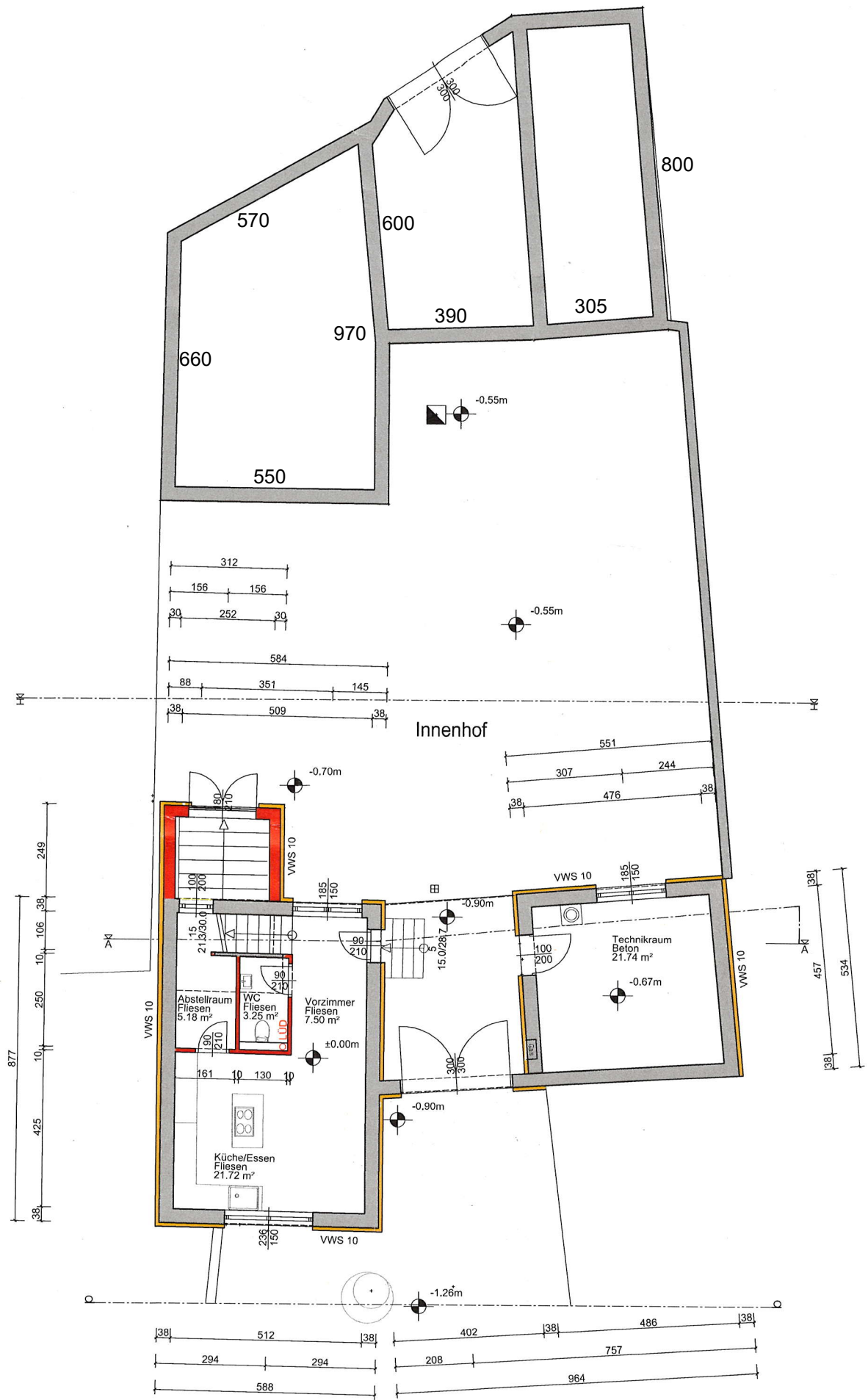
ERDGESCHOSS
