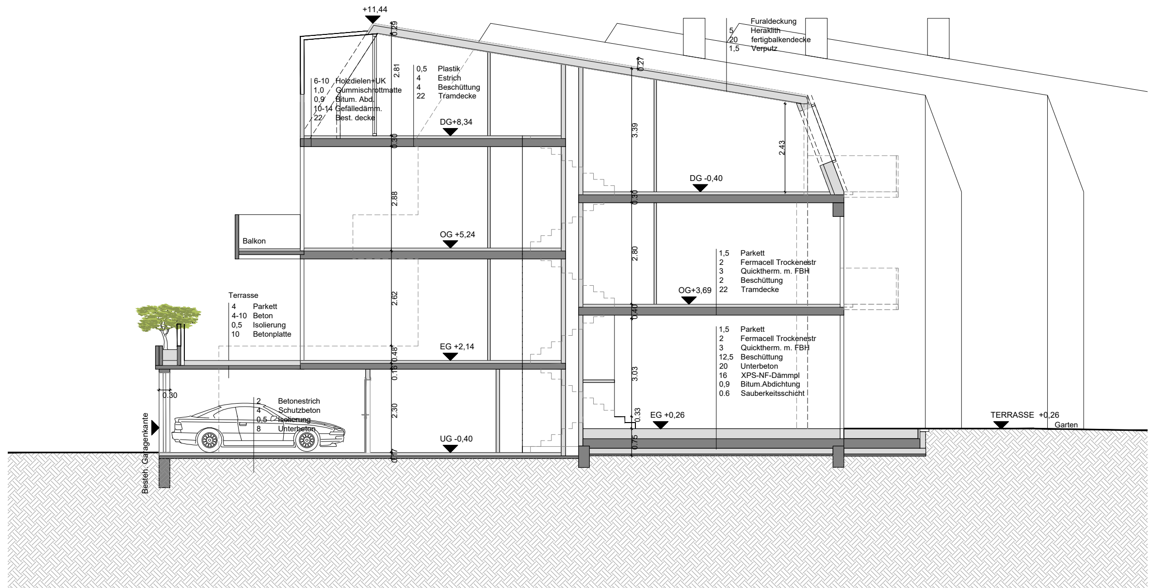
SCHNITT A-A
