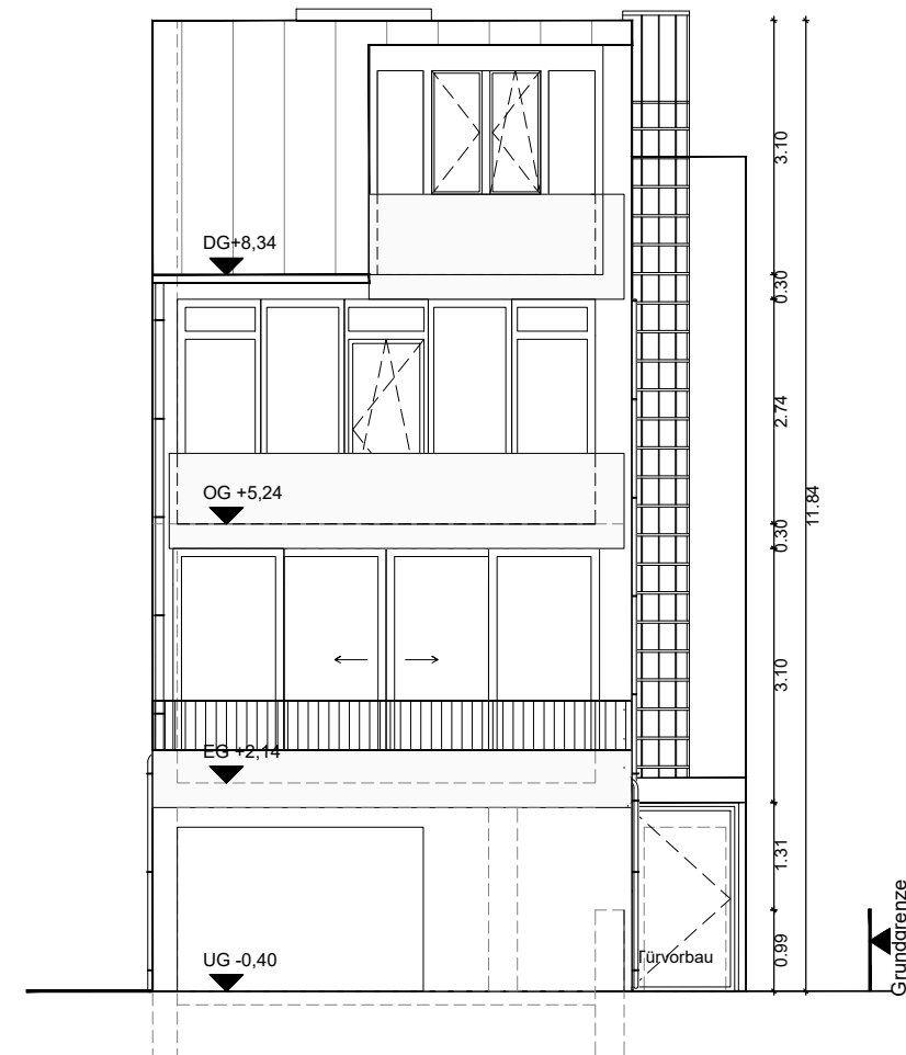
WESTANSICHT
