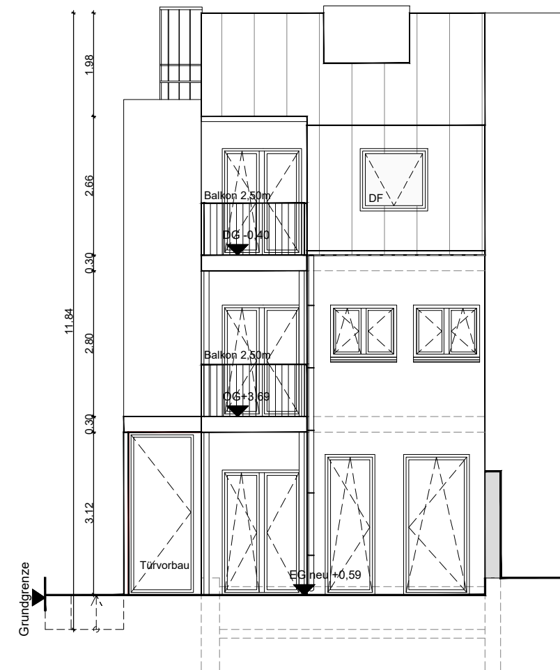
OSTANSICHT
