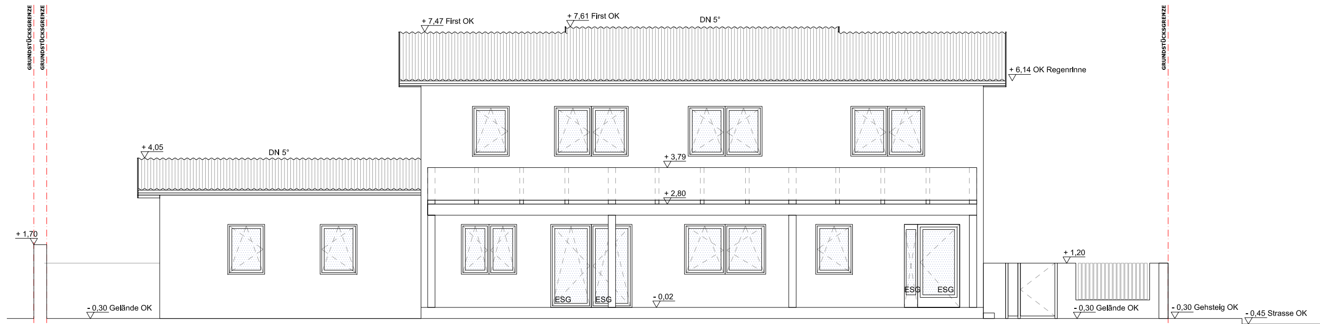
ANSICHT SÜDWEST
