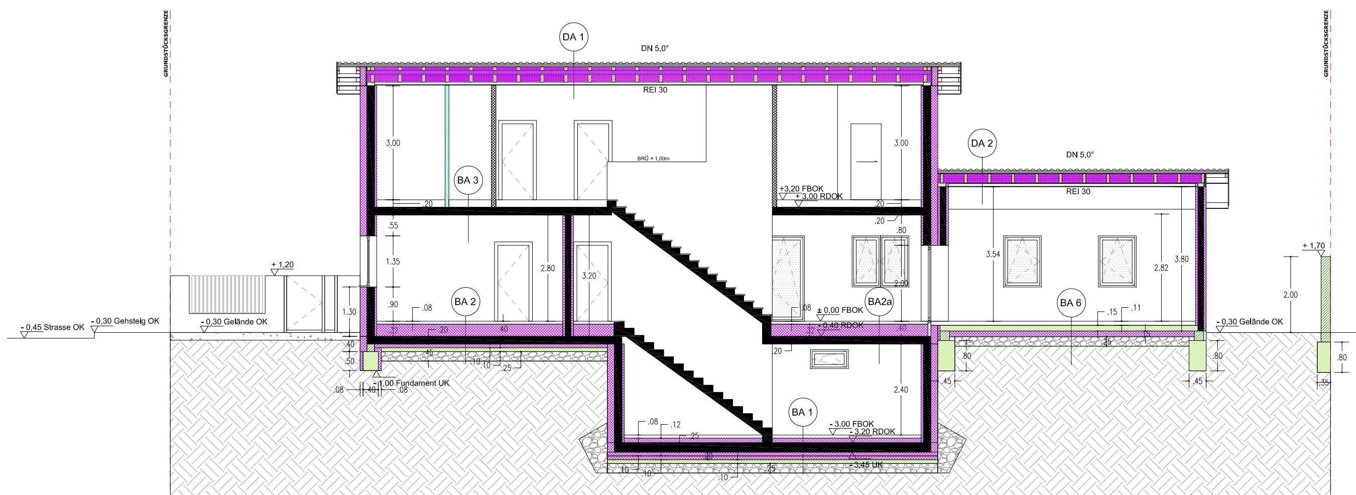
SCHNITT 1
