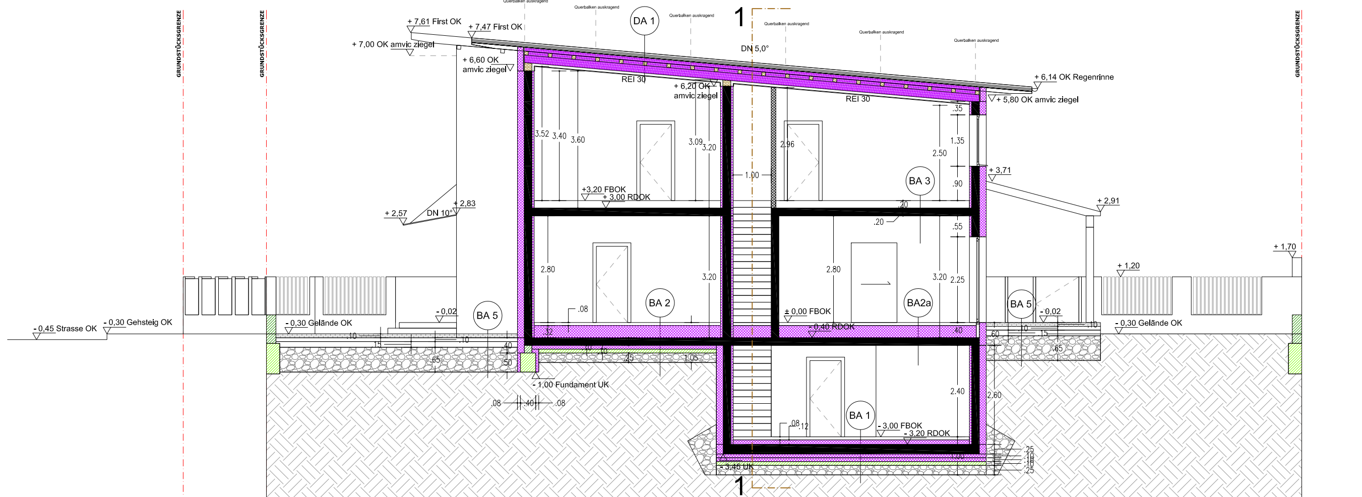
SCHNITT 2
