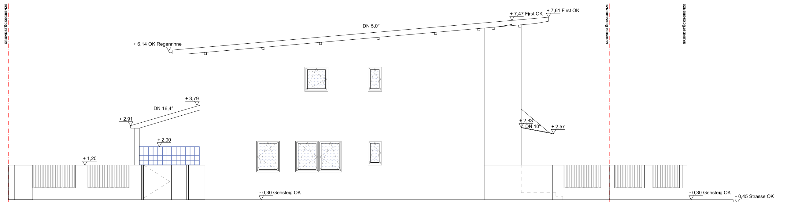
ANSICHT SÜDOST
