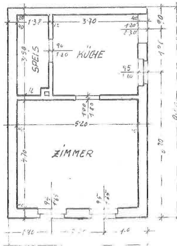
GRUNDRISS (SCHNITT C, D) - 1:100
