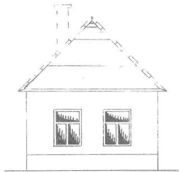
STRASSENANSICHT - 1:100
