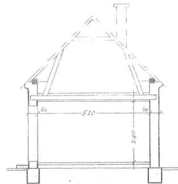
SCHNITT A, B - 1:100
