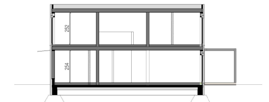
SCHEMATISCHER SCHNITT M 1:300
