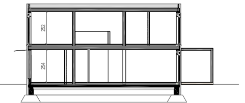
SCHEMATISCHER SCHNITT M 1:300
